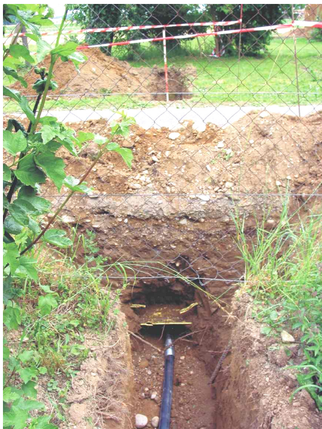
Der TERRA-HAMMER TU 068/75plus SK beim Einlaufen. Er wurde vorgängig mit einem TERRA-Peilstab in Höhe und Neigung ausgerichtet.
